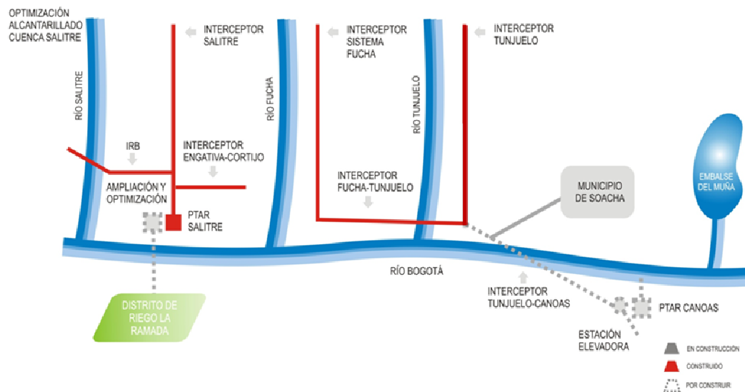
Gráfico 30. Esquema de obras para el Saneamiento del Río Bogotá
