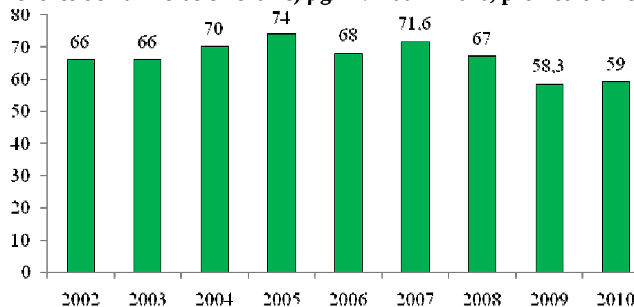
Gráfico 86. Concentración promedio anual del PM10 (niveles de concentración de polvo menores de 10 micras en el aire) \mu\text{g}/\text{m}^3 . 2002 – 2010, promedio directo
